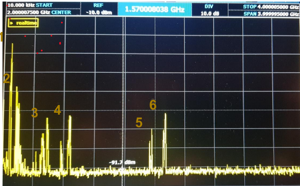
Ilustración 8 Analizador de espectro Fuente: el autor.
