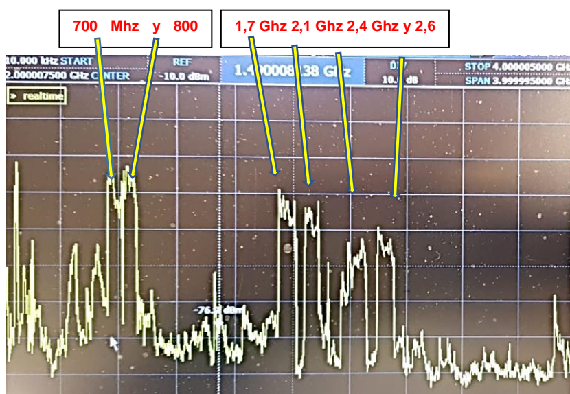
Ilustración 11 Ancho de banda de un de radio bases de teléfonos celulares Fuente: el autor.
